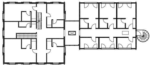
Obergeschoss
